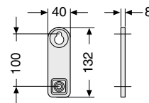
konzola
